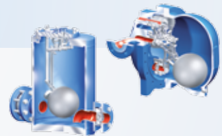
Mechanische Pumpsysteme CONLIFT®, CONA® P
